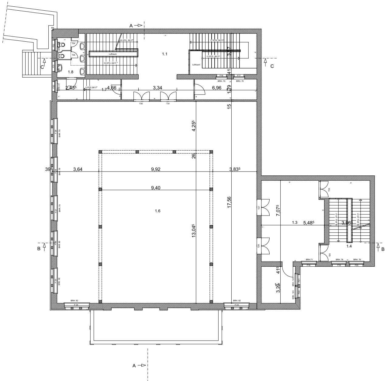
Grundriss Gemeindehaus 1.OG
