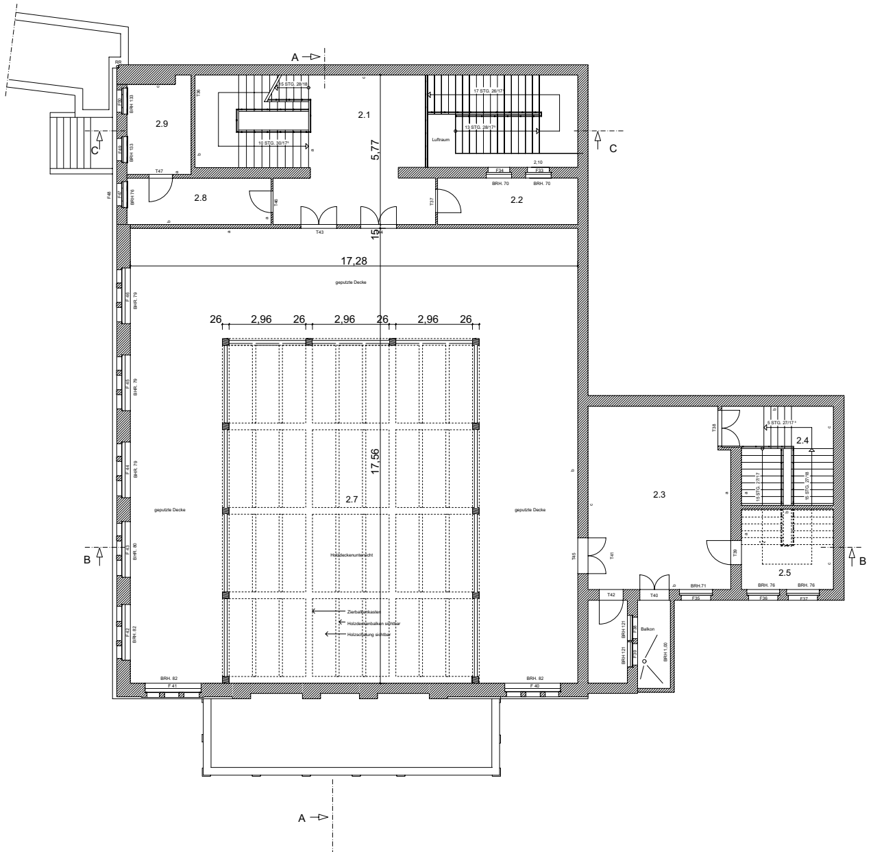
Grundriss Gemeindehaus 2.OG
